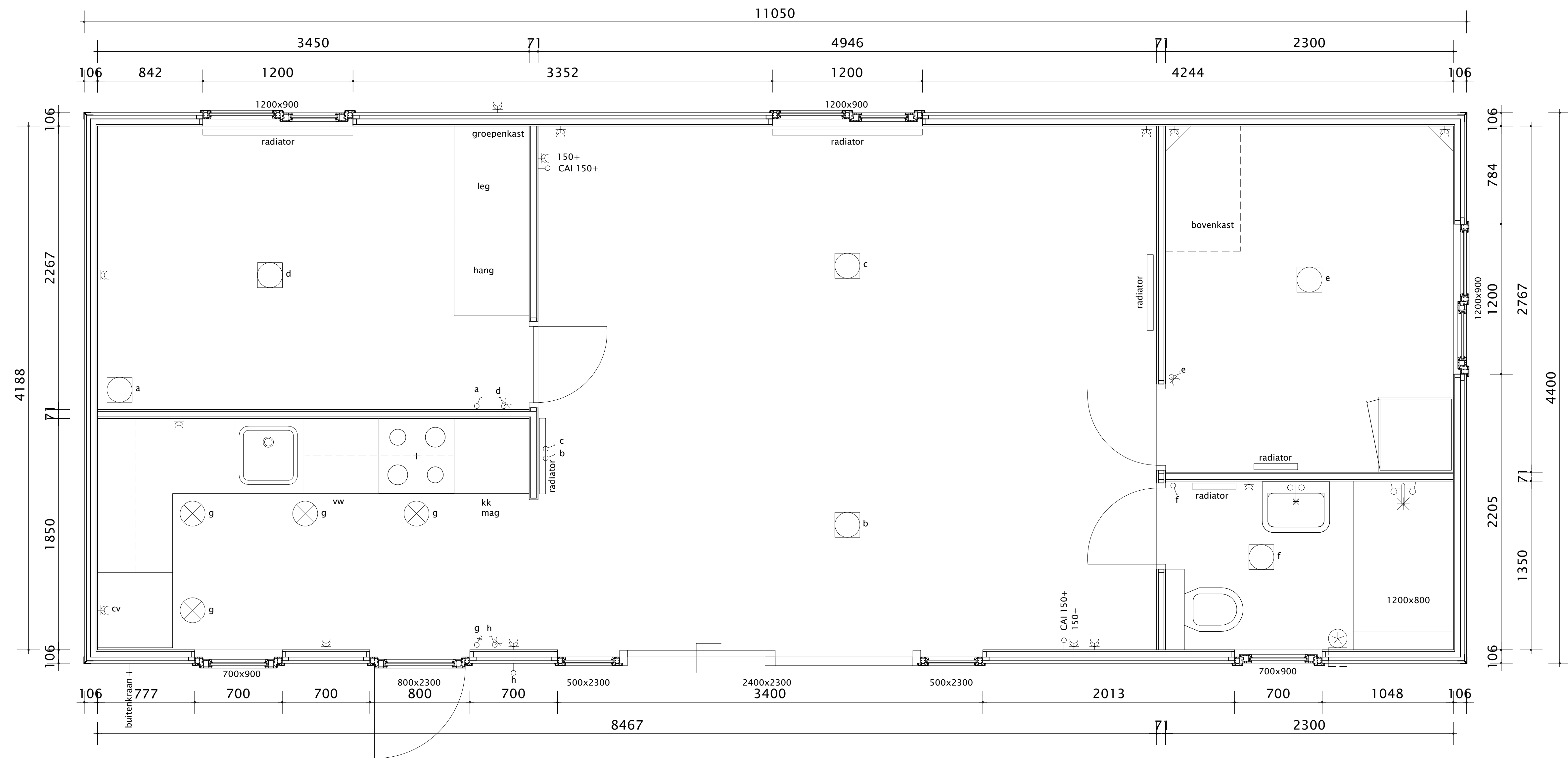
Plattegrond (1:20)
